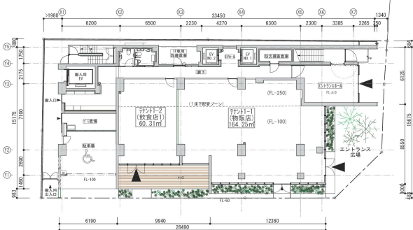
1階平面図 1/200
